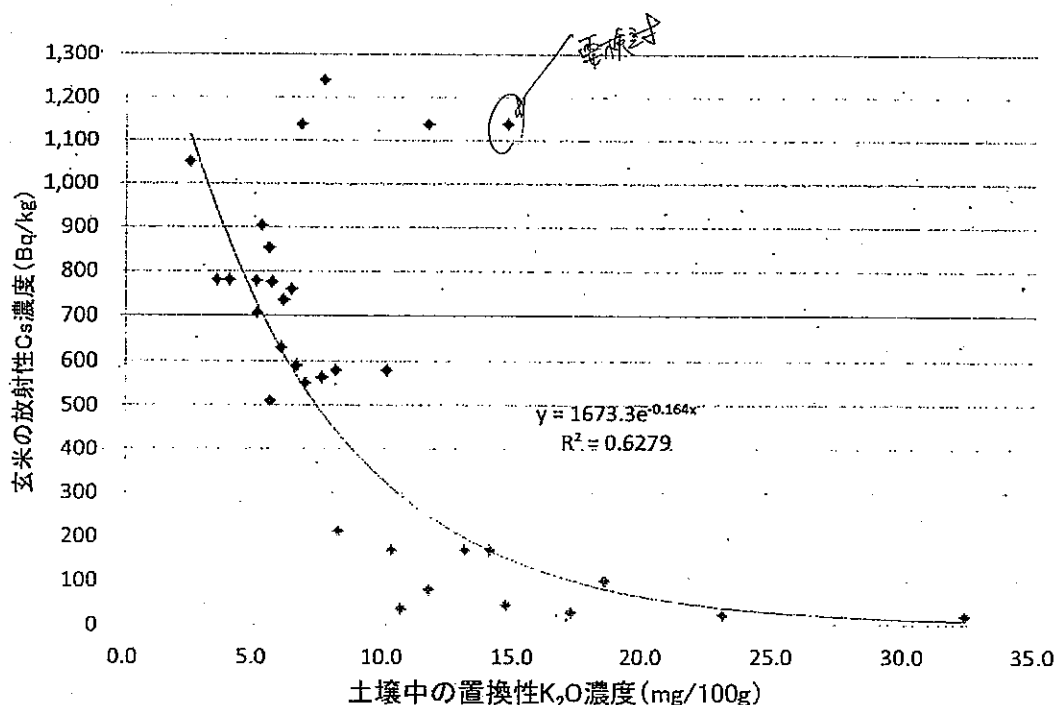
図 4 土壌の置換性カリウム濃度と玄米の放射性セシウム濃度との関係
