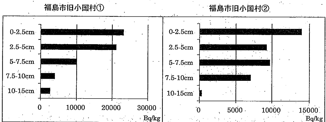
図3 土壌の層別放射性セシウム濃度(福島市旧小国村の2ほ場のデータ)
