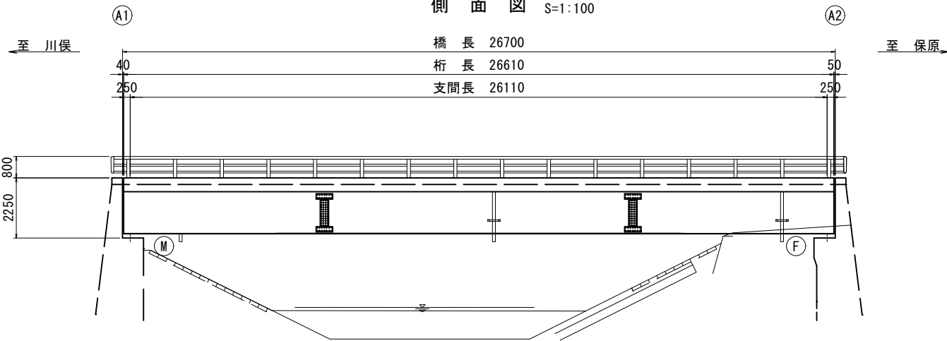
側 面 図 S=1:100
