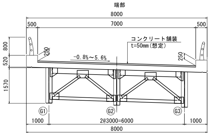
標準断面図 S=1:50
