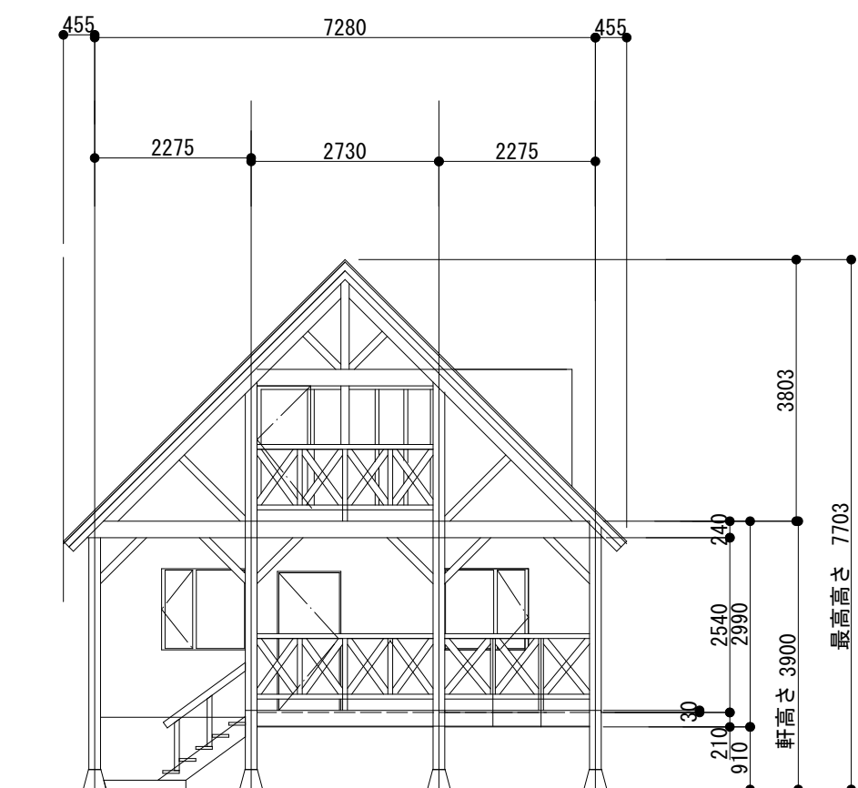
南側立面図 1 : 100
