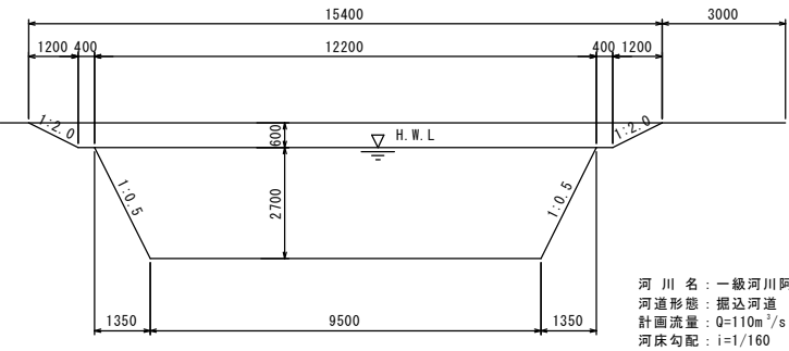
計画河川断面図 S=1:100
