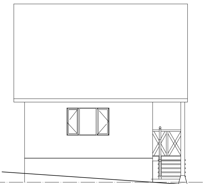
西側立面図 1 : 100
