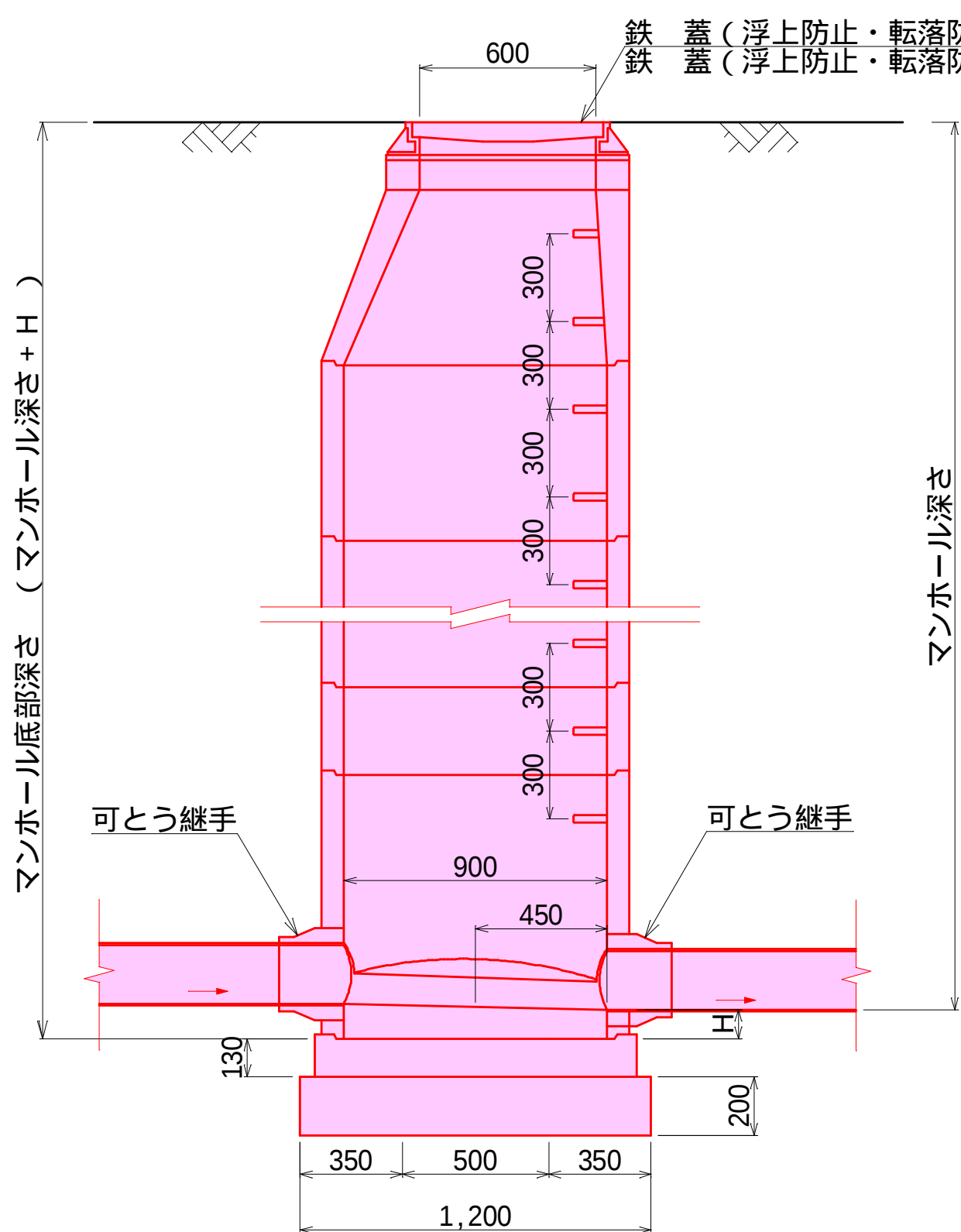
縦 断 面 図
