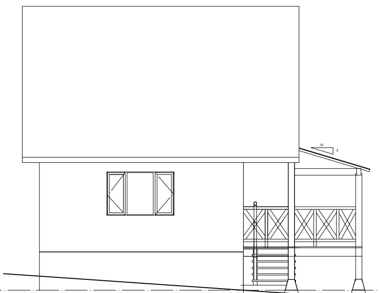
西側立面図 1 : 100
