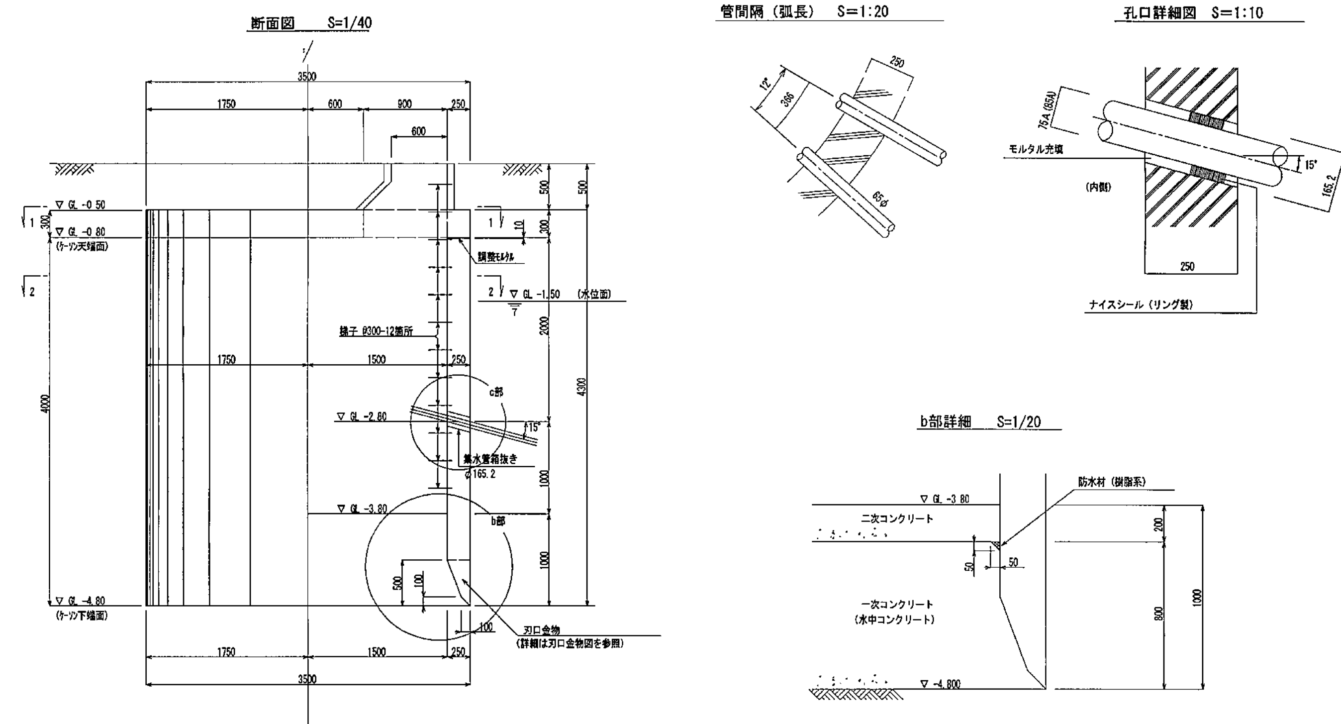
孔口詳細図 S=1:10
