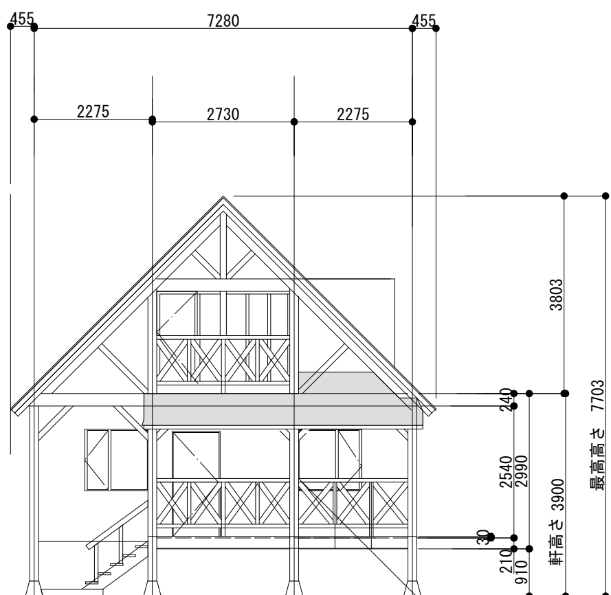
南側立面図 1 : 100
