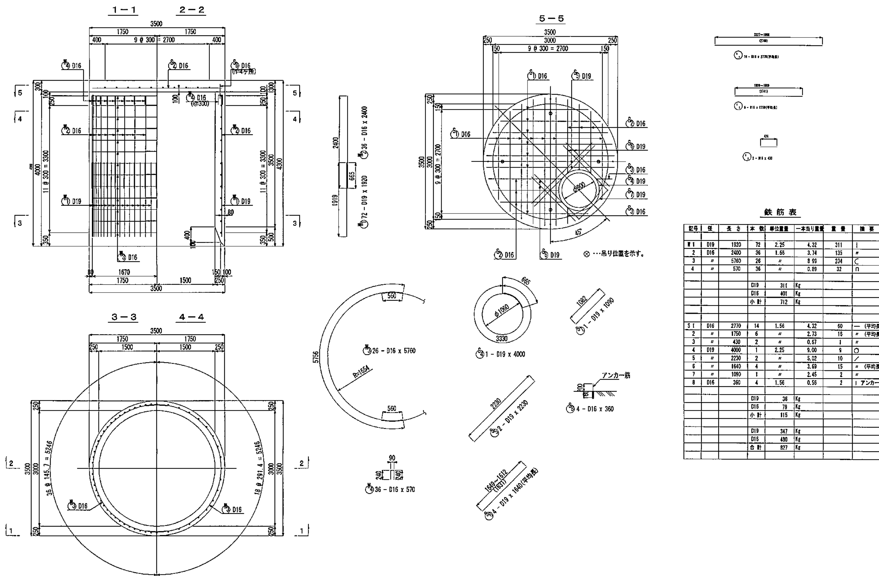
保原採熱水槽配筋図 S=1/60
