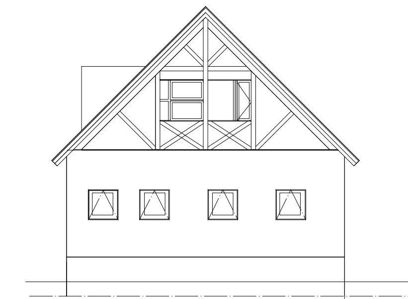
北側立面図 1 : 100
