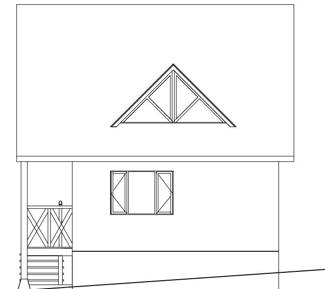
東側立面図 1 : 100
