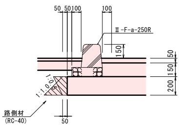
a 部詳細図 S=1:20
