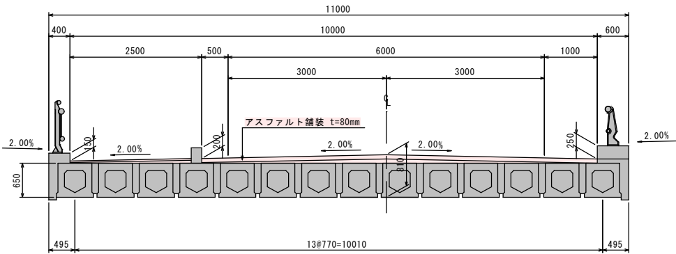
上部工断面図 S=1:50
