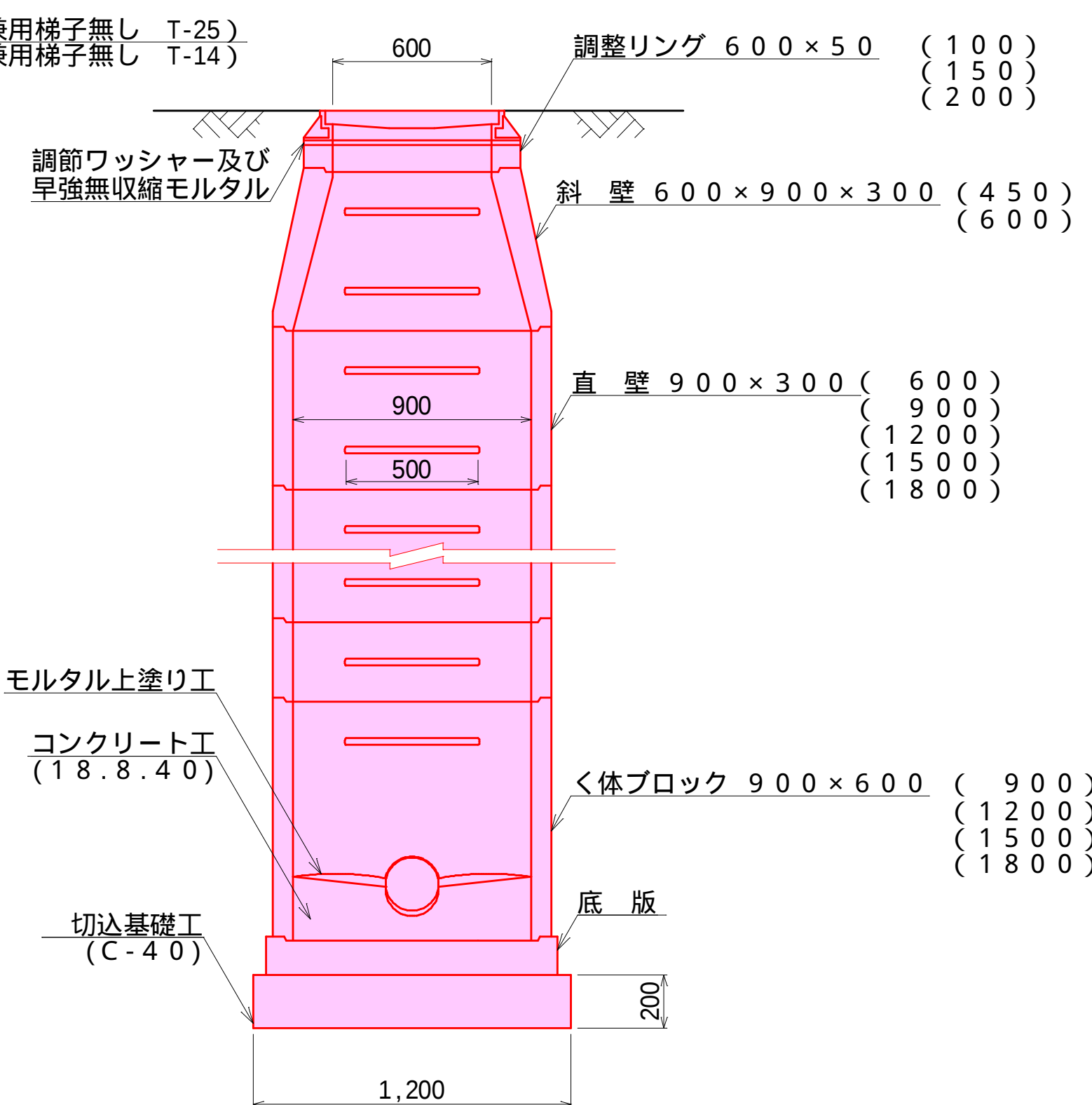
横 断 面 図
