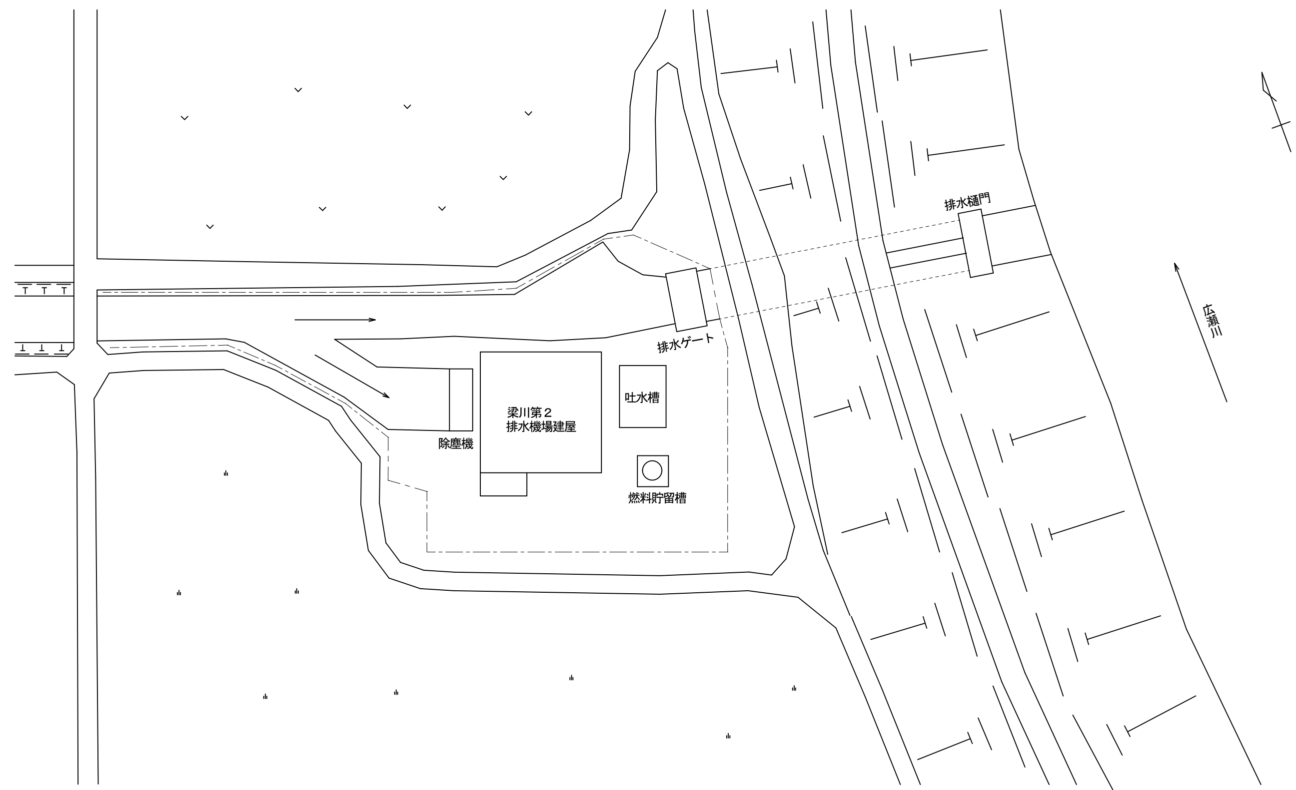
平面図 S=1:500
